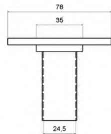
Zur Aufnahme eines M25-Installationsrohres
